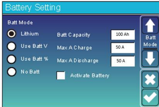
Configuración 1 Batería
